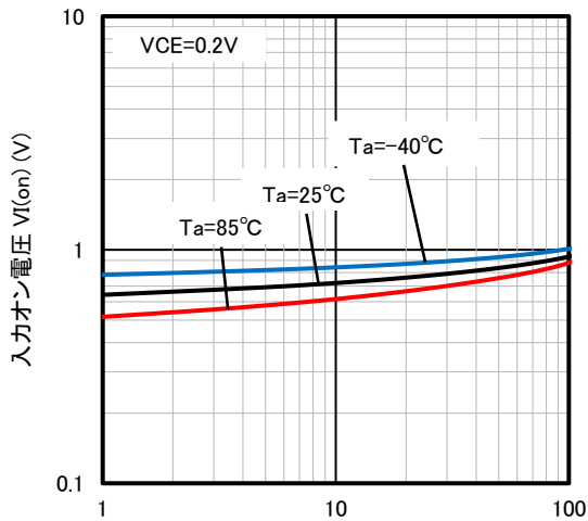
コレクタ電流 I_C (mA)
